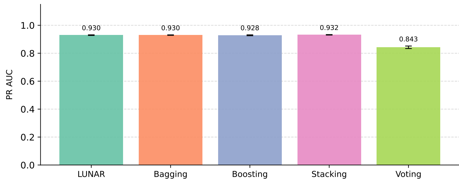
UNSW-NB15
