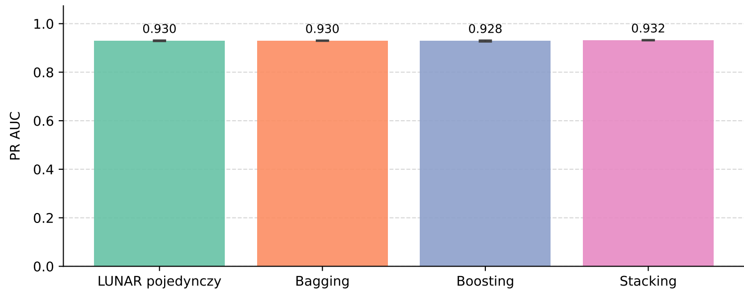
UNSW-NB15
