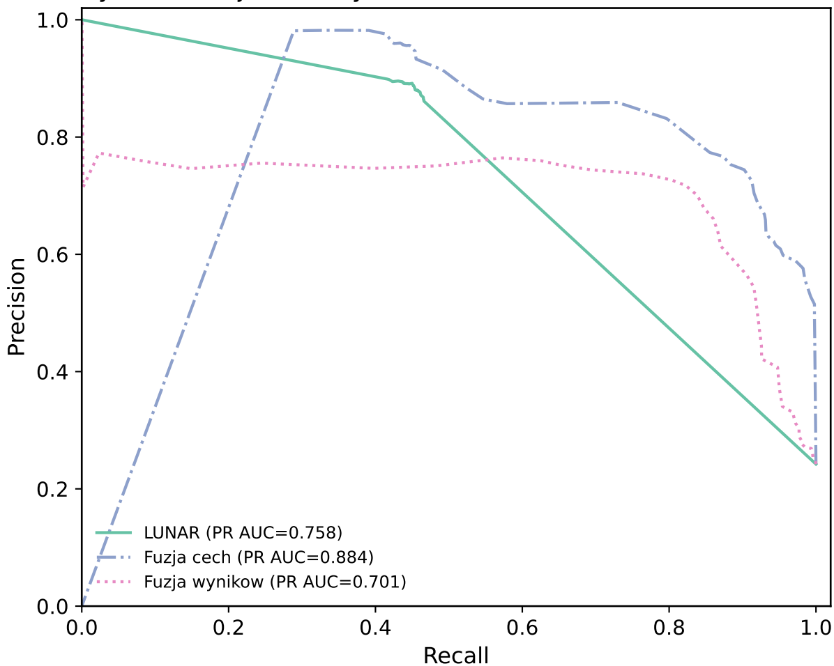
Krzywe PR: fuzja cech/wynikow vs modele bazowe -- CICIDS 2017
