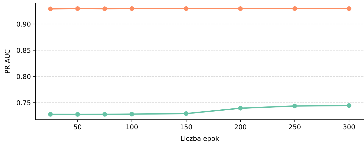
Jakość detekcji (PR AUC)
