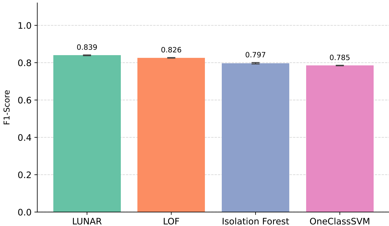
F1 modeli pojedynczych (próg standardowy) — UNSW-NB15
