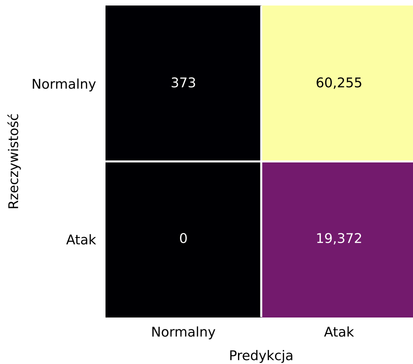
OneClassSVM
