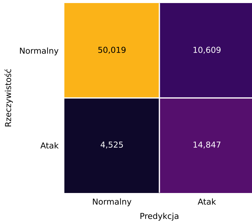
LOF
