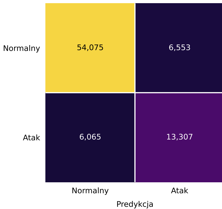
LUNAR
