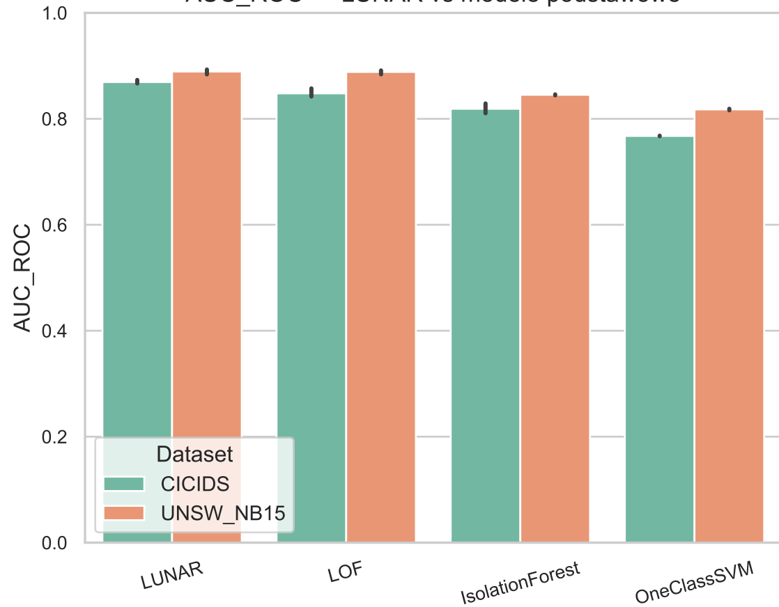
AUC_ROC — LUNAR vs modele podstawowe
