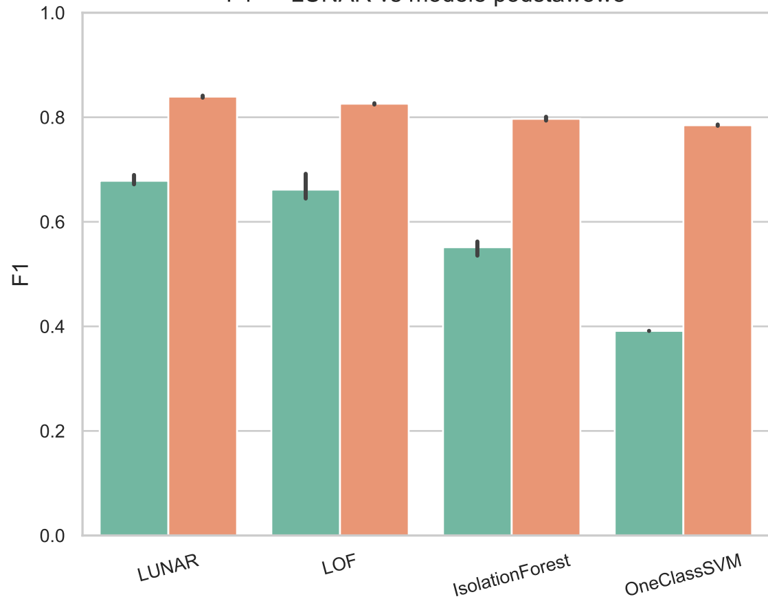
F1 — LUNAR vs modele podstawowe
