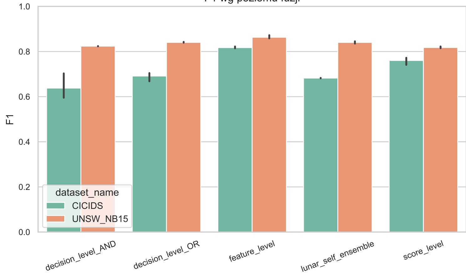
F1 wg poziomu fuzji
