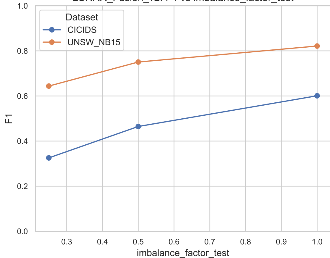
LUNAR_Fusion_v2: F1 vs imbalance_factor_test
