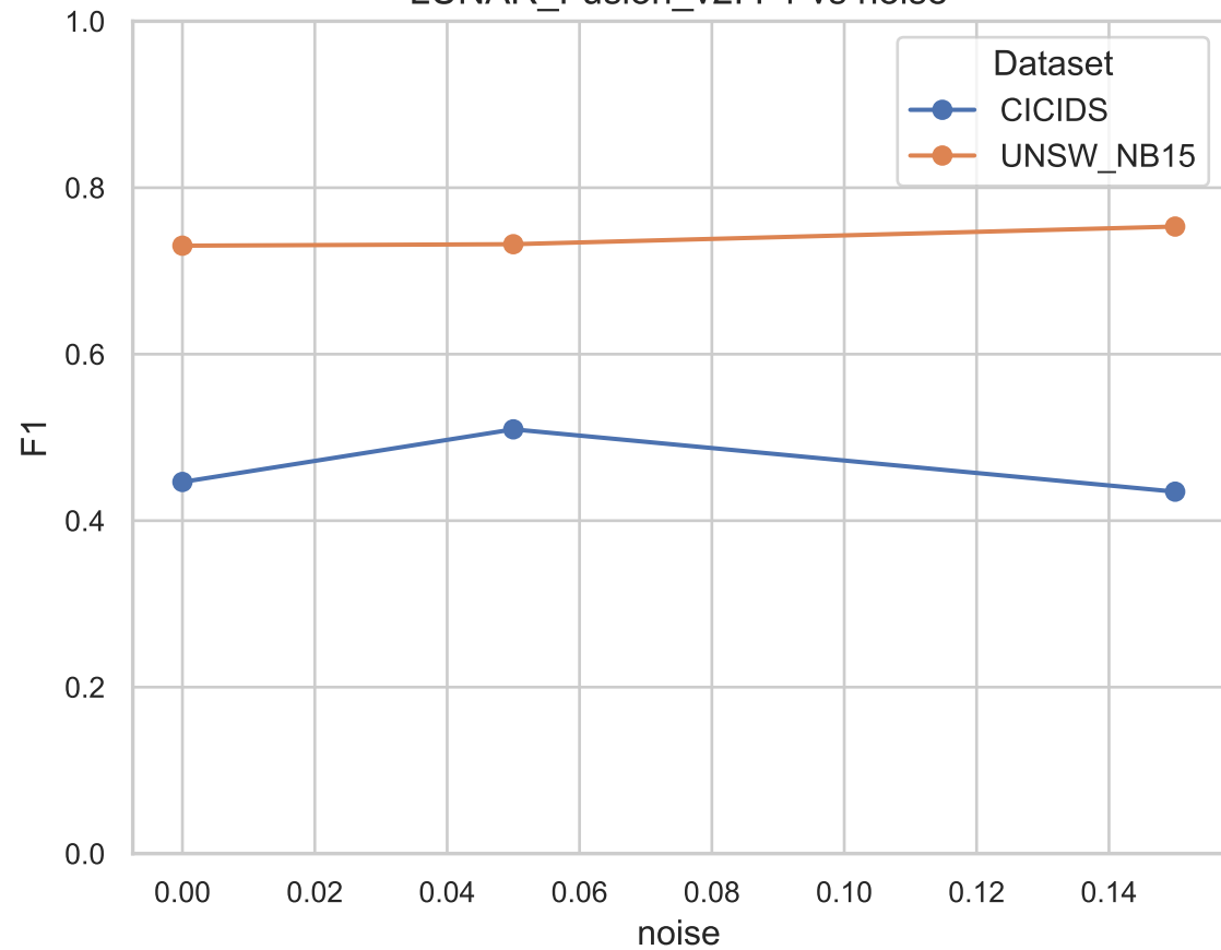
LUNAR_Fusion_v2: F1 vs noise
