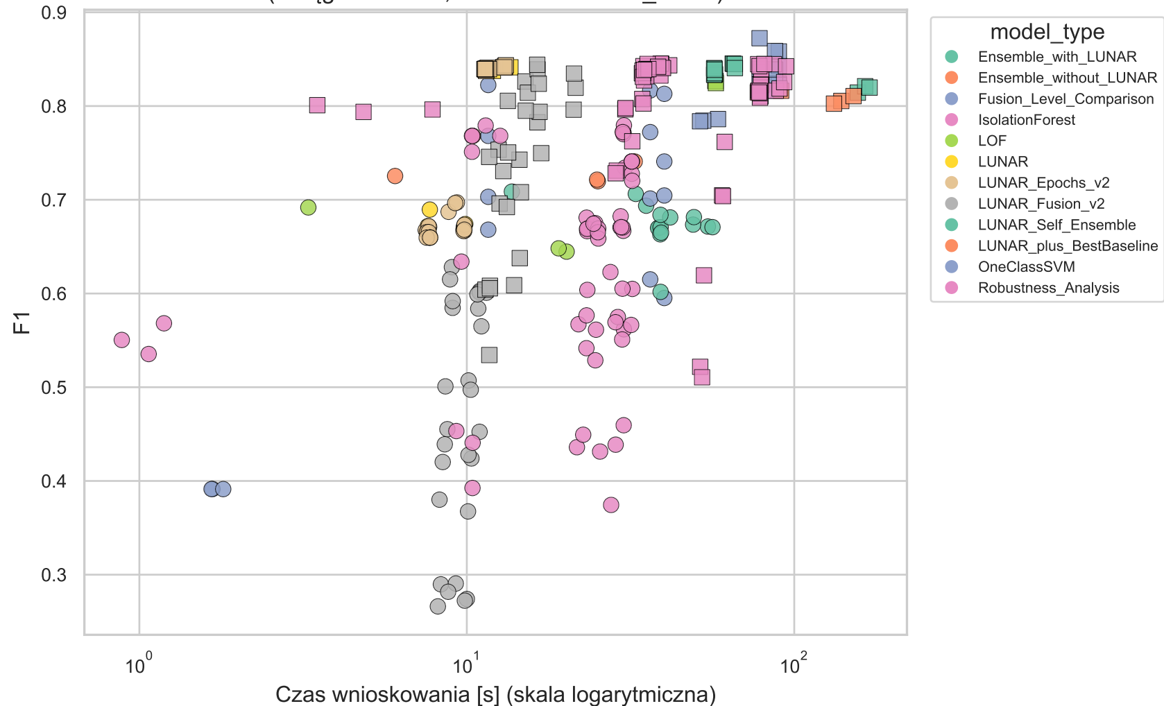
Trade-off: jakość (F1) vs czas wnioskowania (okrąg = CICIDS, kwadrat = UNSW_NB15)
