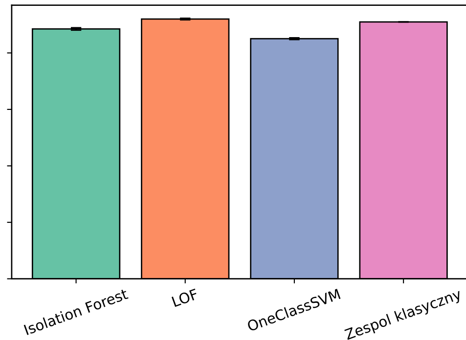
UNSW-NB15
