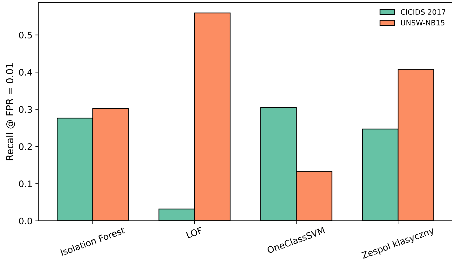
Czułosc modeli klasycznych i zespołu klasycznego przy FPR \leq 1\%
