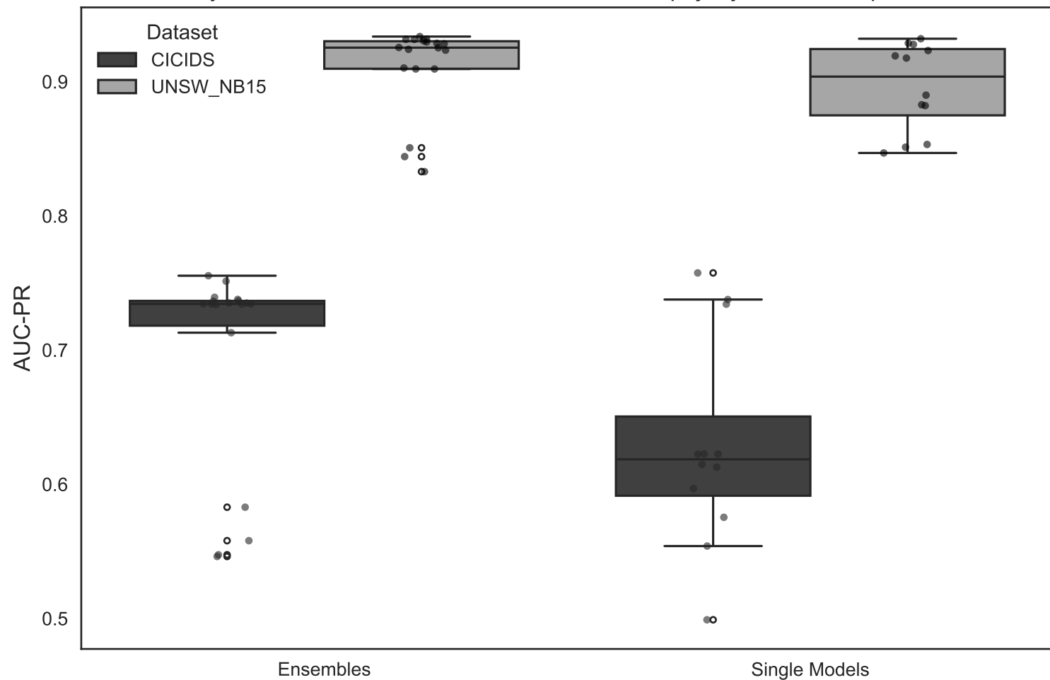
Wykres 2. Stabilnosc i skutecznosc: modele pojedyncze vs zespolowe
