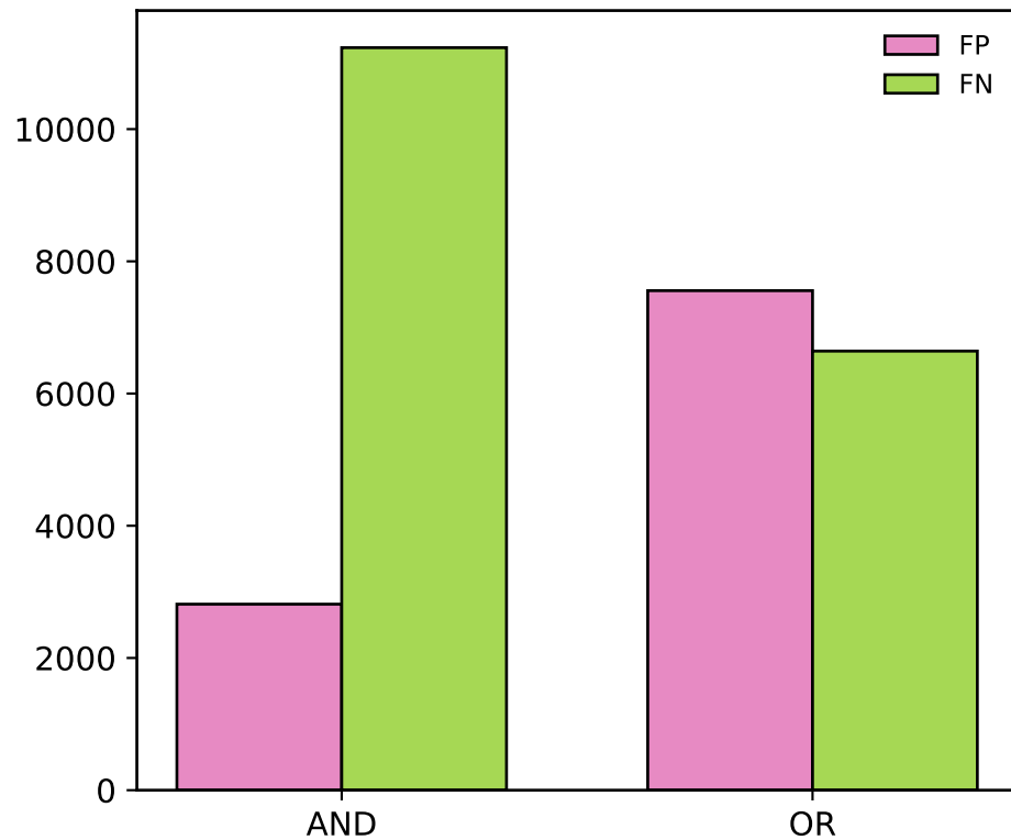
UNSW-NB15
