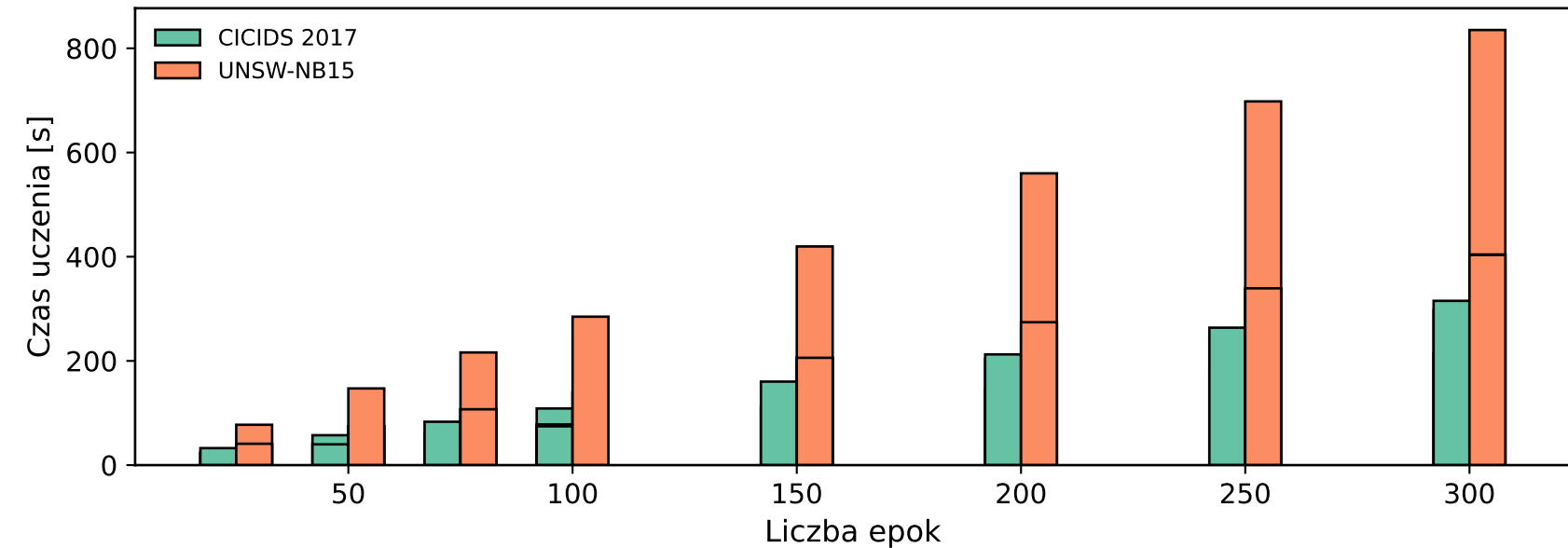
Czas uczenia w funkcji liczby epok
