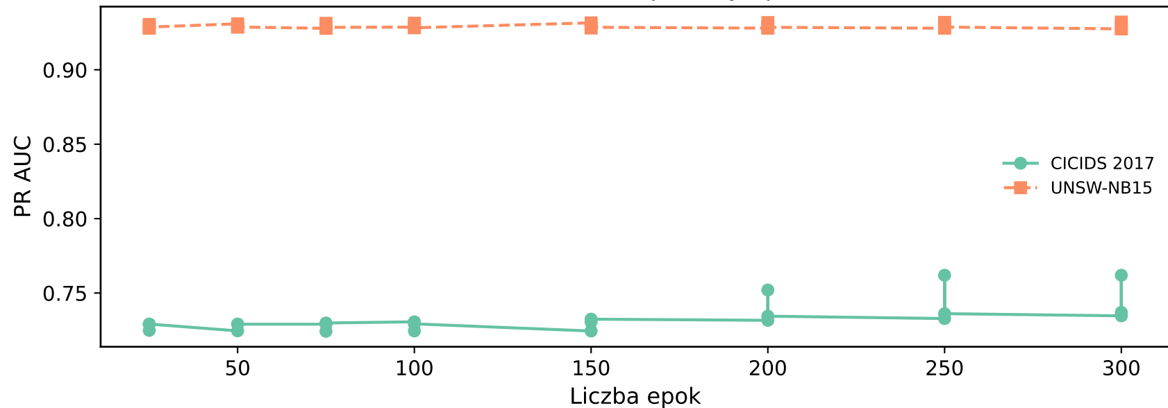
PR AUC w funkcji liczby epok
