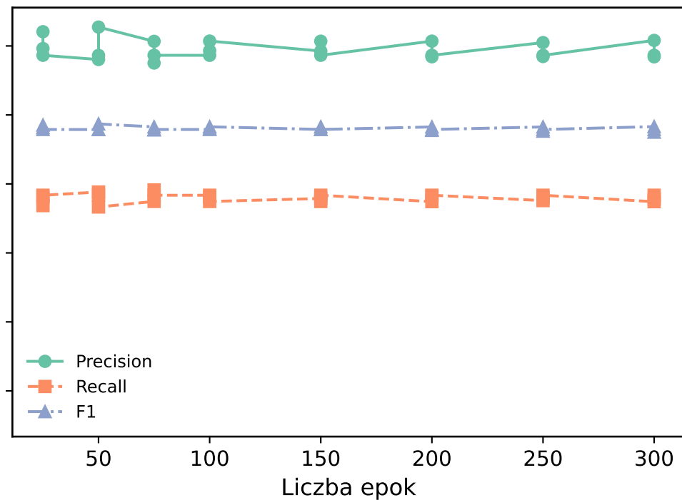
UNSW-NB15
