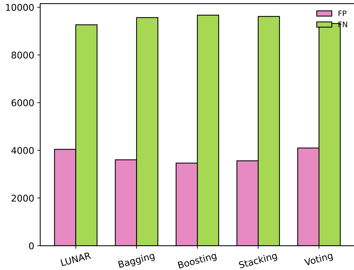
UNSW-NB15
