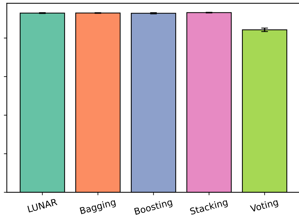
UNSW-NB15
