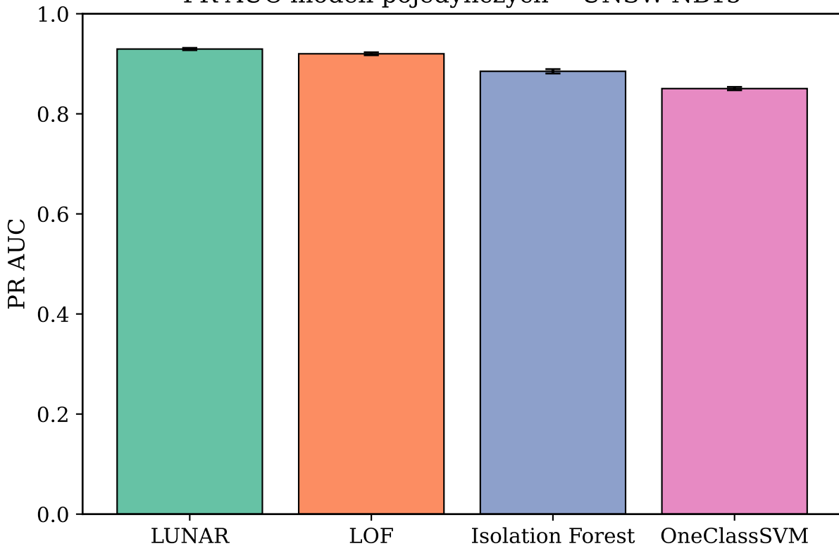
PR AUC modeli pojedynczych -- UNSW-NB15
