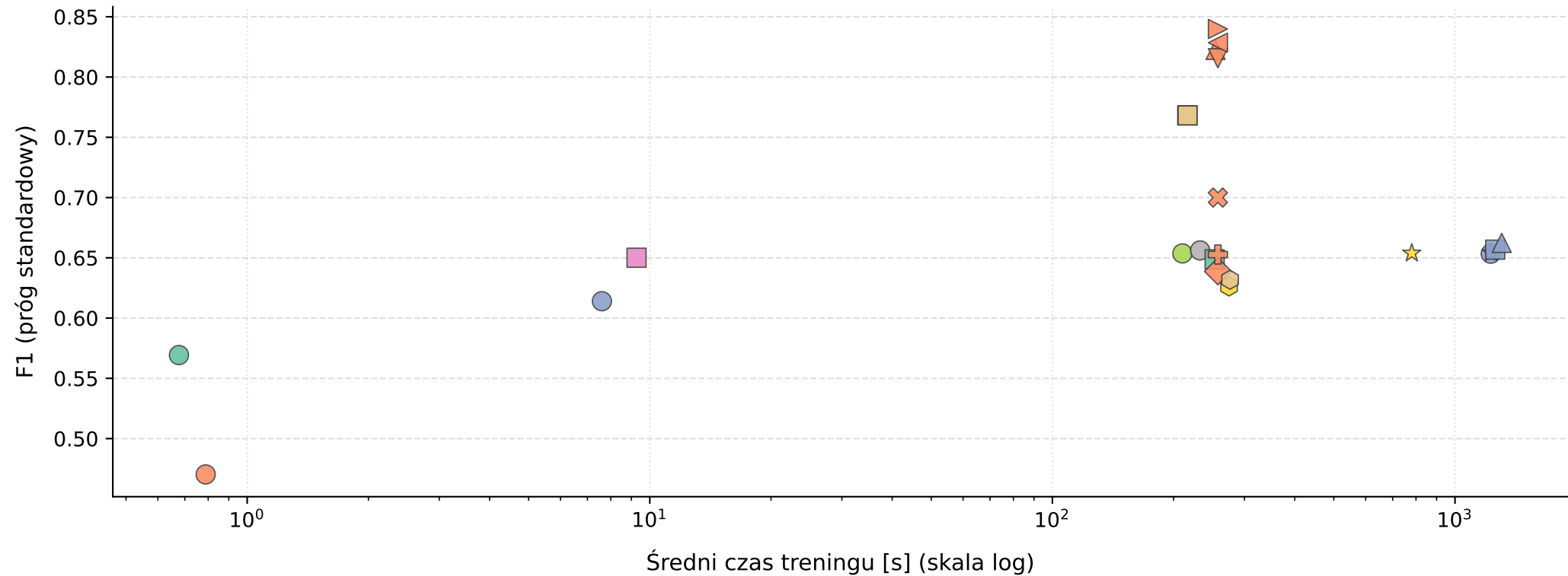
Koszt treningu vs jakość detekcji — CICIDS2017, Run 1
