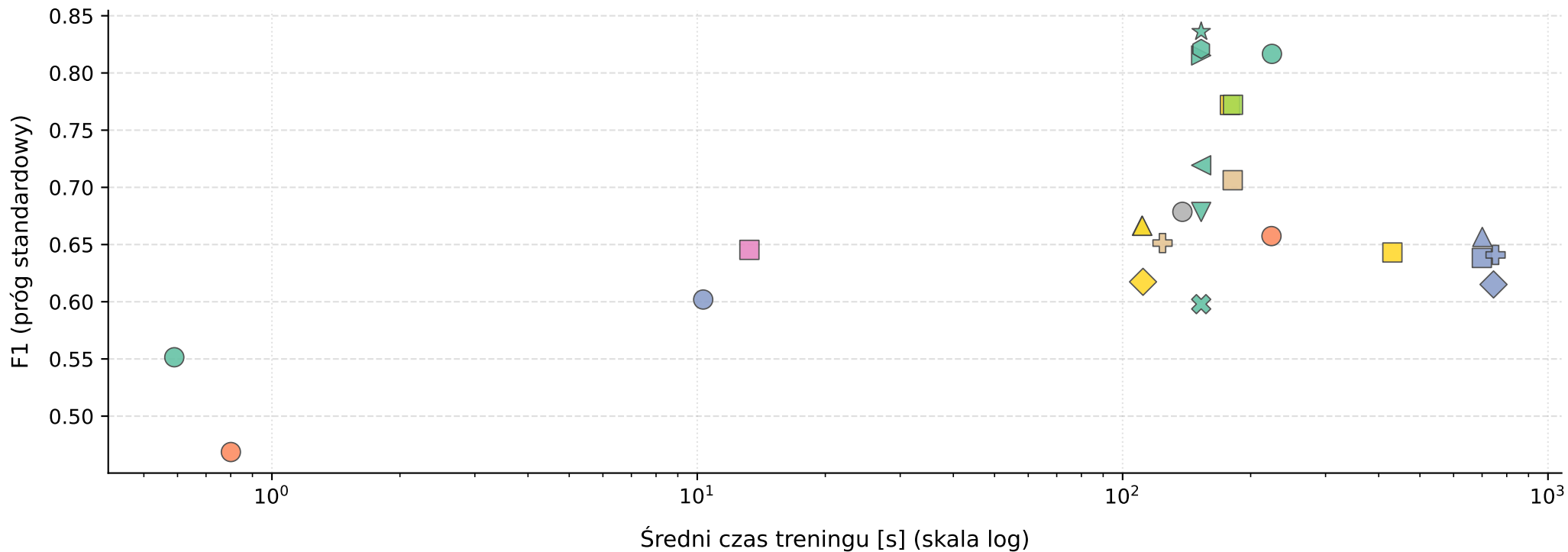
Koszt treningu vs jakość detekcji — CICIDS2017, Run 2
