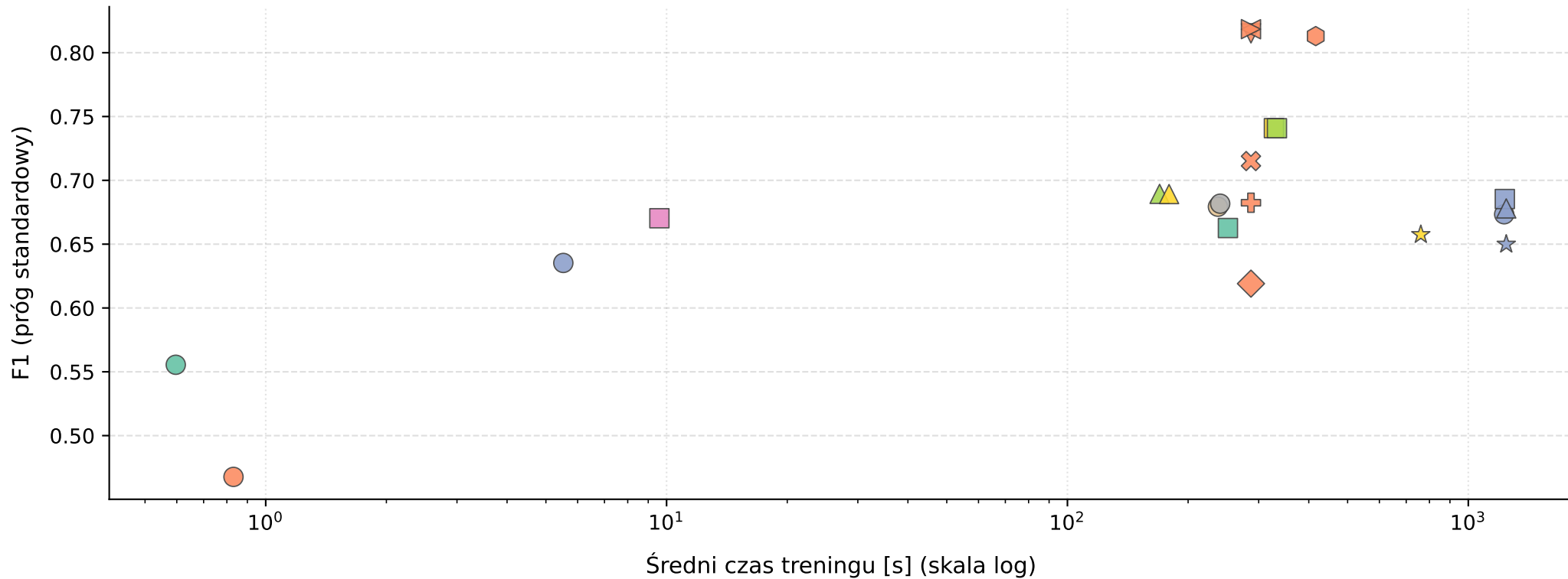
Koszt treningu vs jakość detekcji — CICIDS2017, Run 3
