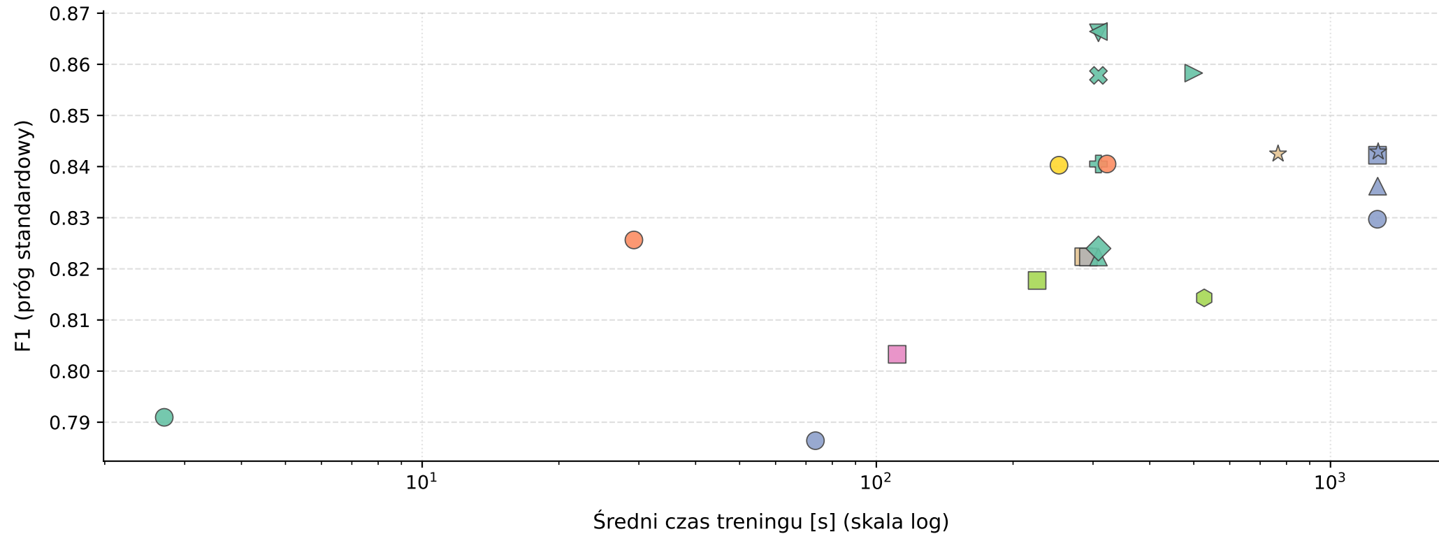
Koszt treningu vs jakość detekcji — UNSW-NB15, Run 1
