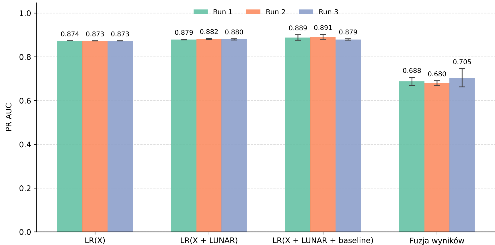
PR AUC wariantów fuzji z ciągłym wynikiem anomalii — CICIDS2017
