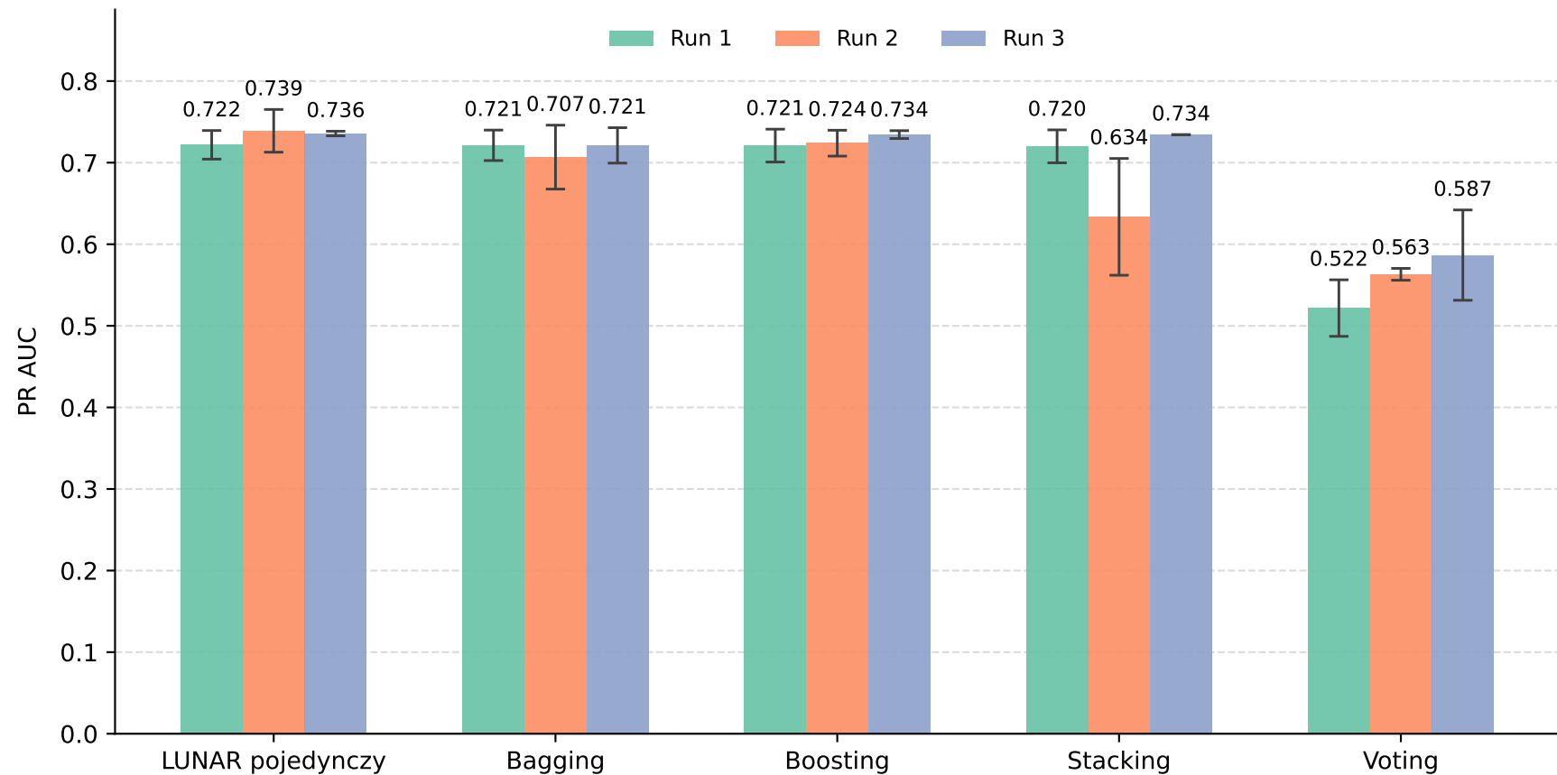
PR AUC: LUNAR pojedynczy i zespoły homogeniczne — CICIDS2017
