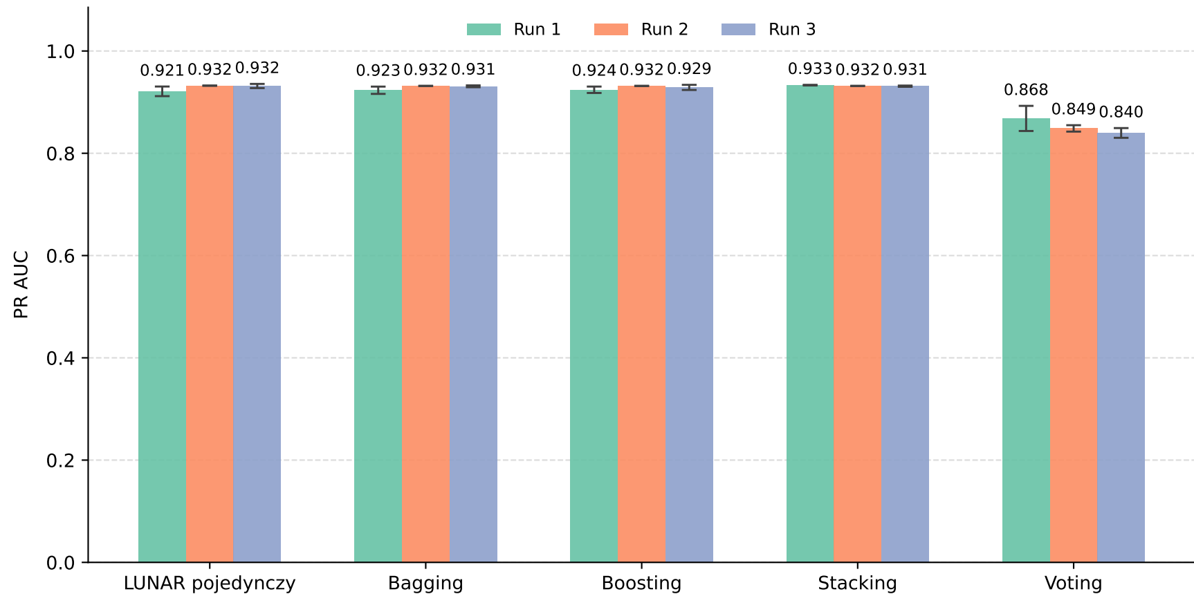
PR AUC: LUNAR pojedynczy i zespoły homogeniczne — UNSW-NB15
