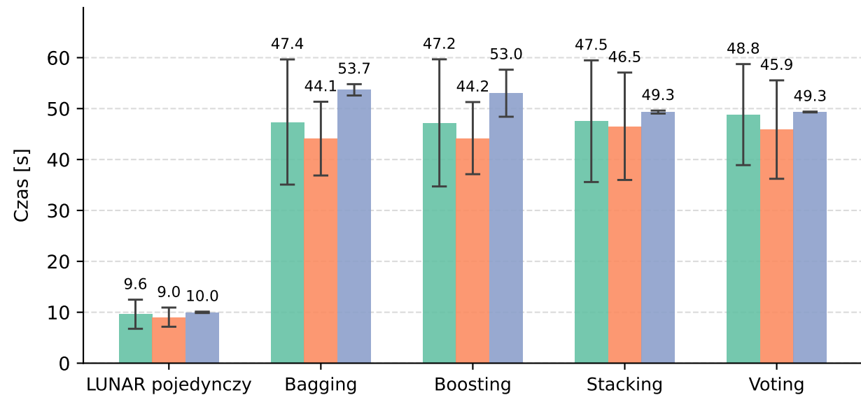
Czas wnioskowania
