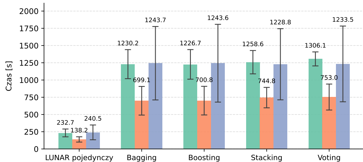
Czas uczenia
