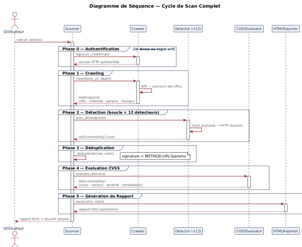
Figure 3.4. Diagramme de séquence — cycle de scan complet
