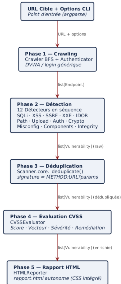
Figure 3.1. Architecture en pipeline du scanner de vulnérabilités
