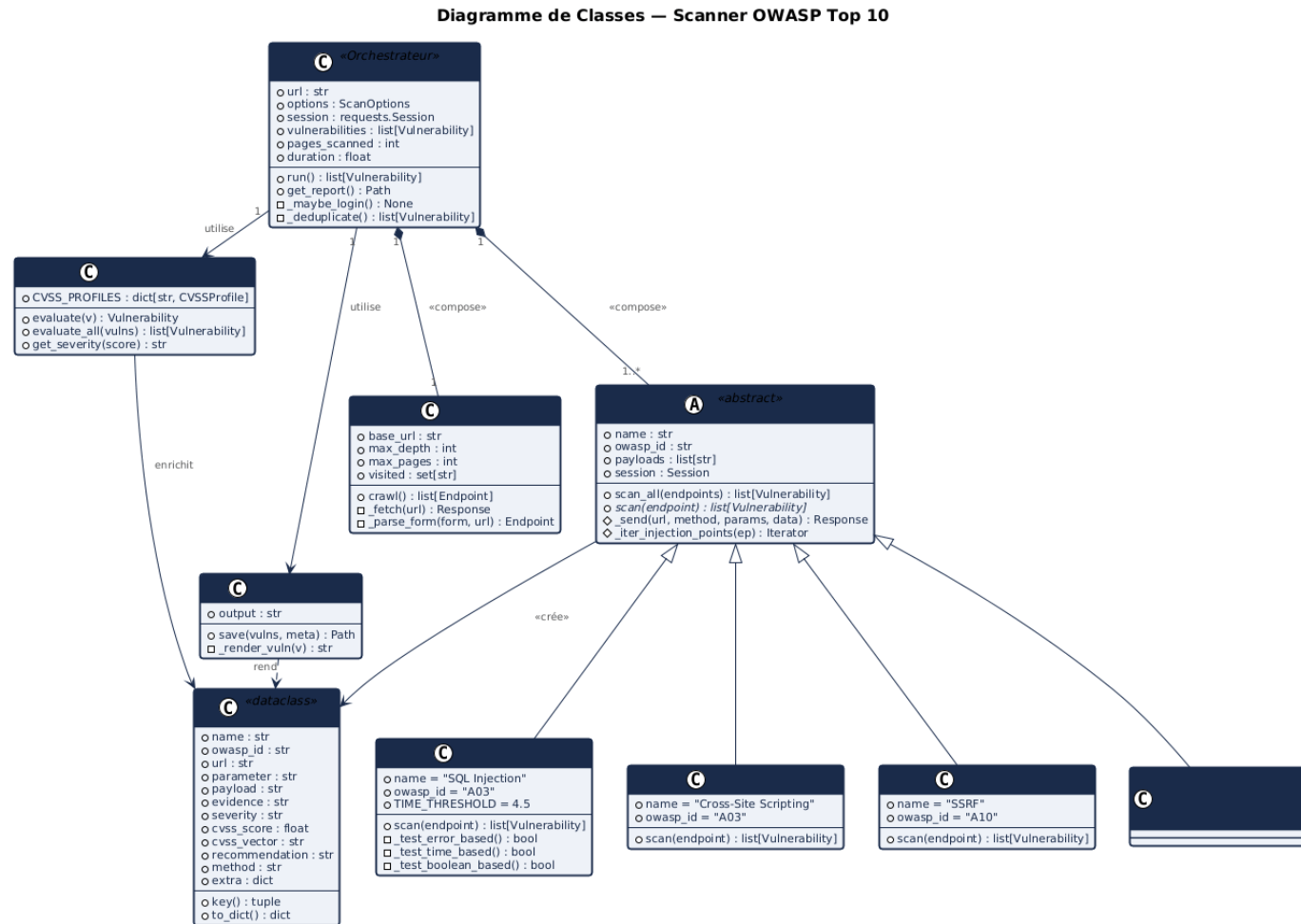
Figure 3.3. Diagramme de classes complet du scanner
