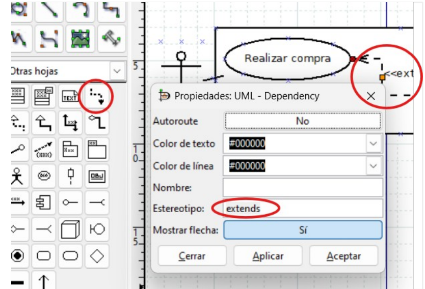
Propiedades de la relación «extend» en DIA: estereotipo "extends"
