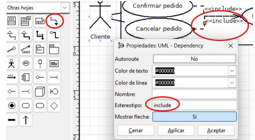
Propiedades de la relación «include» en DIA: estereotipo "include" y flecha activada
