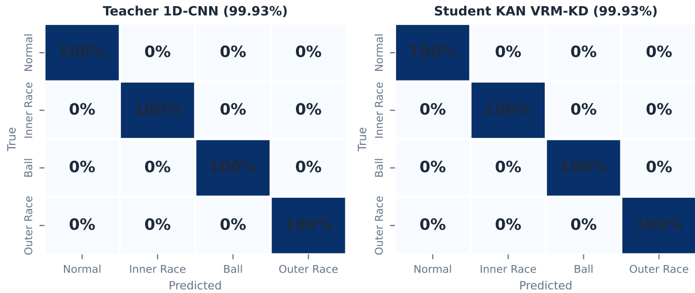
图 6. 混淆矩阵。教师 1D-CNN（左，99.93%）和 VRM-KD 下的 KAN 学生（右，99.93%）在 CWRU 保留测试集（2,743 样本）上。两模型在所有四个故障类别上均实现近乎完美分类。
