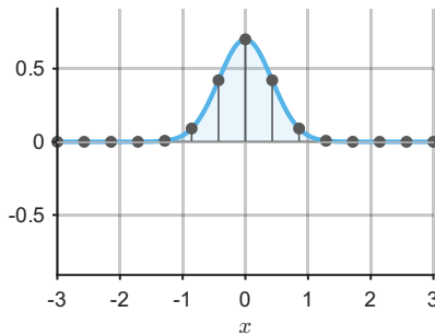
(e) RBF-KAN ( \sigma=0.6 )
