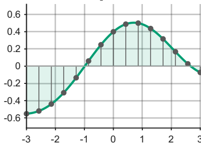
(e) RBF-KAN ( \sigma=0.6 )
