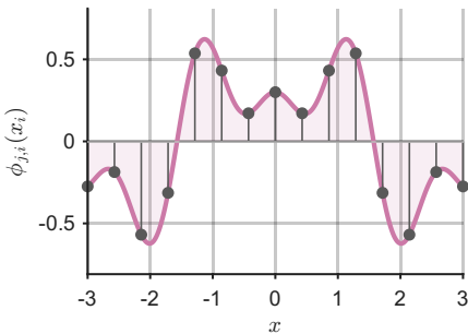
(d) ChebyKAN (deg. 5)
