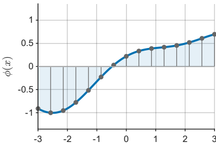
(d) ChebyKAN (deg 5) M_2=3.12
