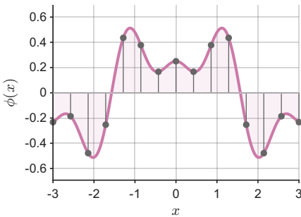
(d) ChebyKAN (deg 5) M_2=3.12
