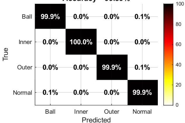
Student KAN [28,16,4] Accuracy = 99.89%
