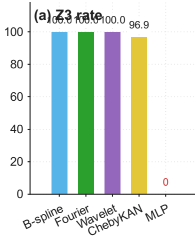
Z3-verifiable (%)
