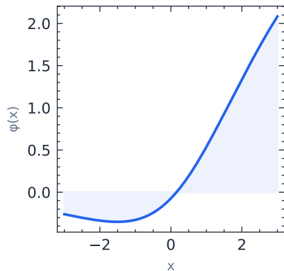
\phi[13 \rightarrow 5]
