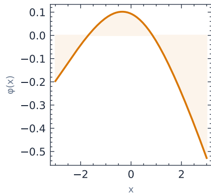
\phi[27 \rightarrow 15]
