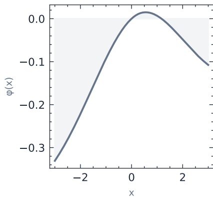
\phi[13 \rightarrow 5]
