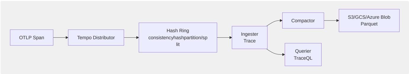
图15-6 Grafana Tempo 架构：无索引设计
