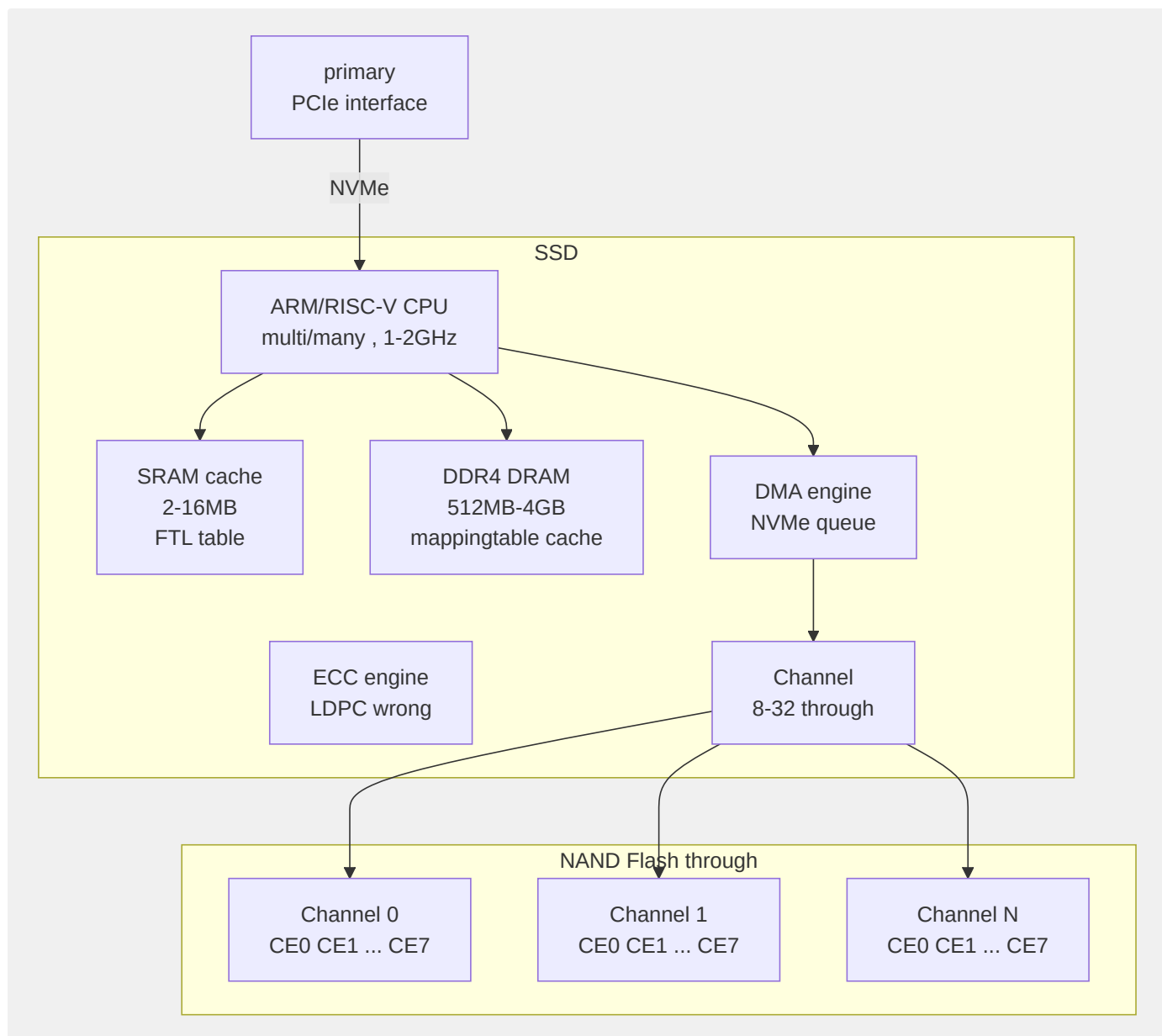
图6-6 SSD 控制器架构
