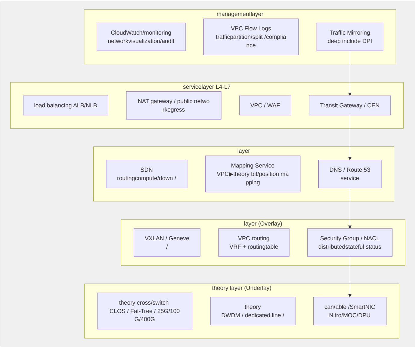
图7-1 云网络五层参考模型
