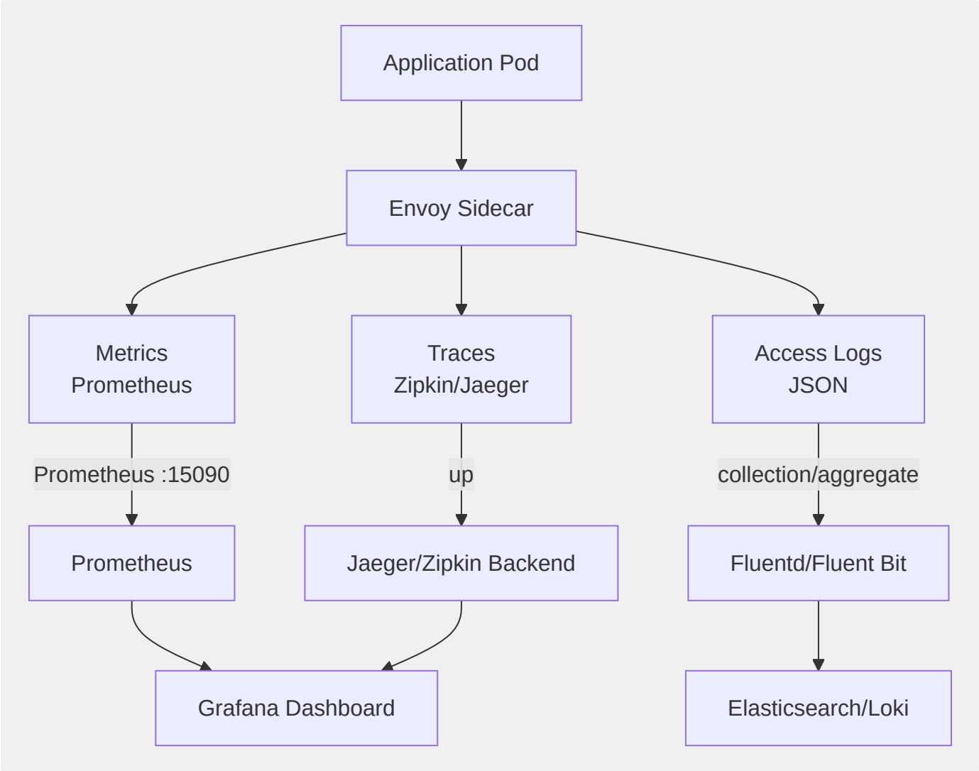
图10-9 Sidecar 中的可观测性数据生成管道
