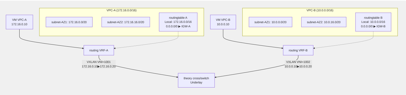
图7-3 VPC 隔离：VRF + VXLAN 实现多租户隔离
