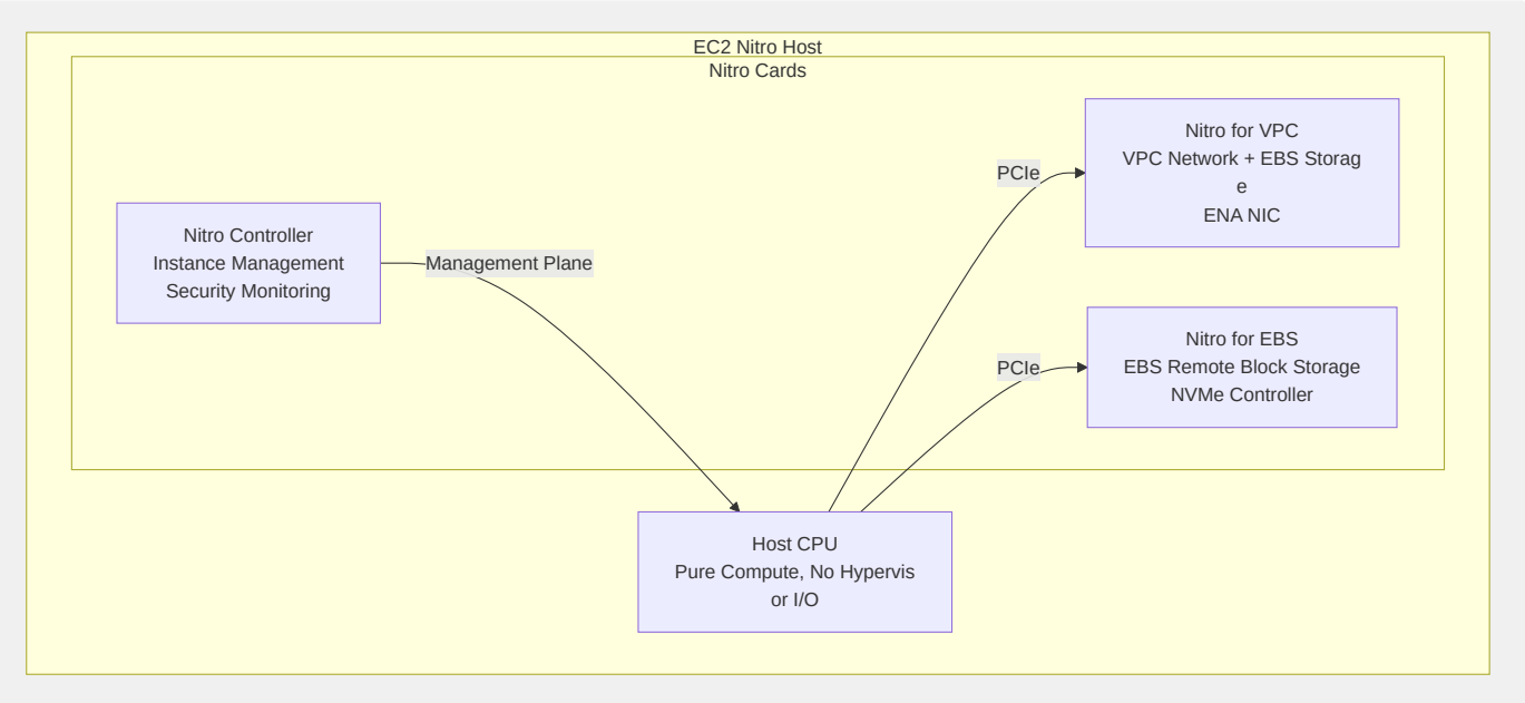
图2-13 AWS Nitro 系统的三卡分离架构
