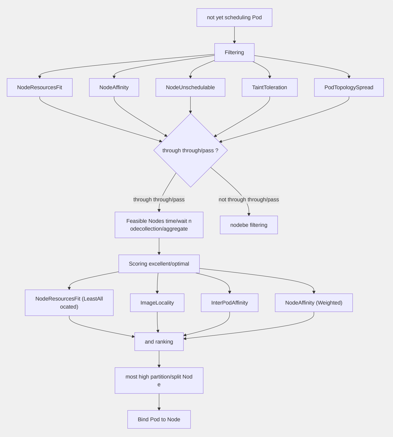
图9-4 kube-scheduler 双阶段调度流程
