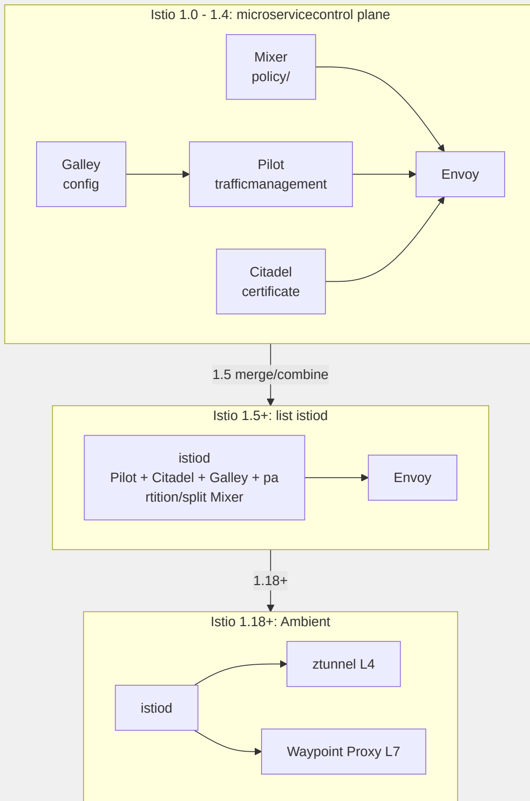
图10-4 Istio 控制面架构的三代演进
