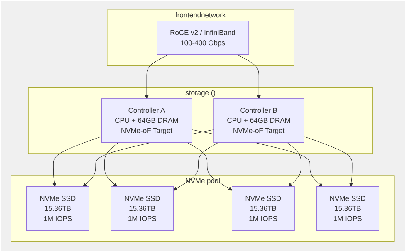
图6-22 NVMe-oF 全闪存阵列架构
