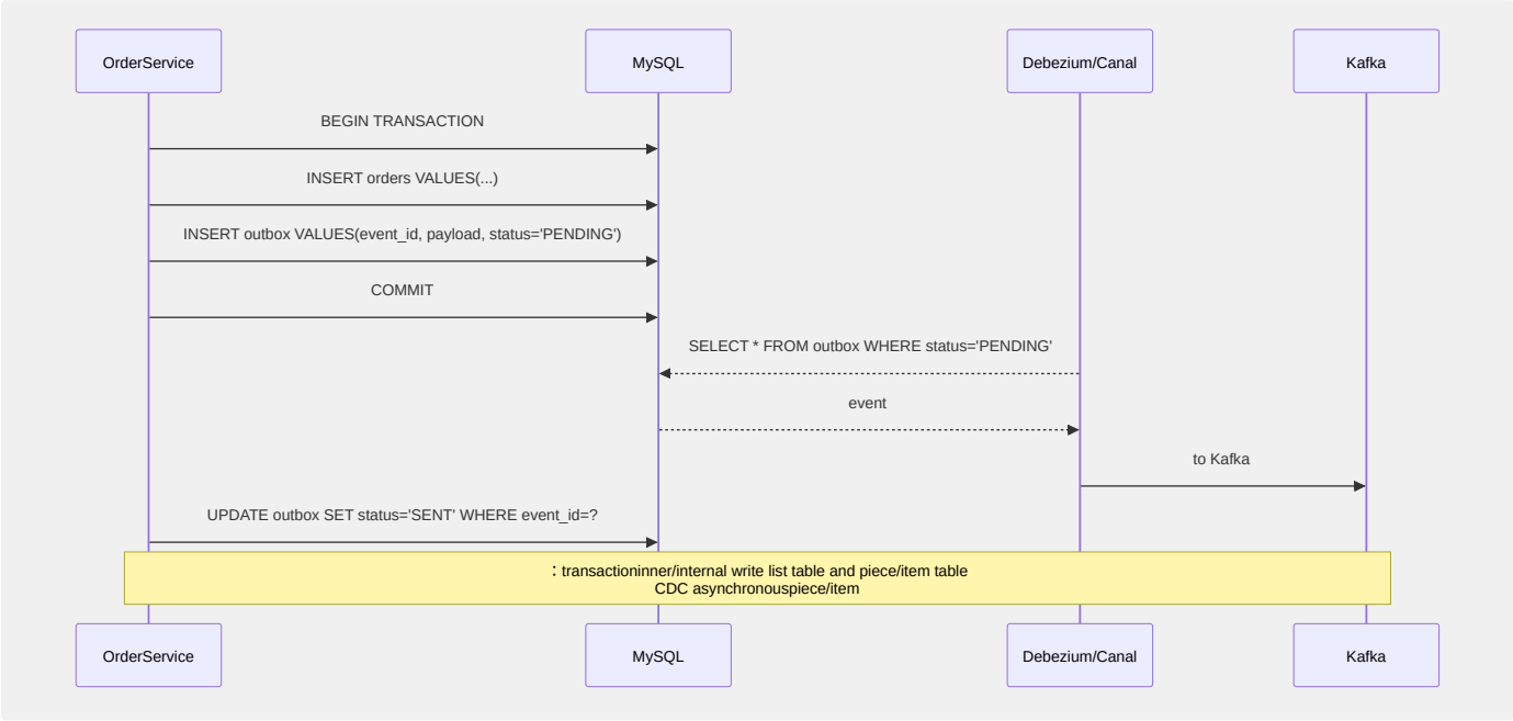
图12-12 Outbox Pattern 事务一致性保障
