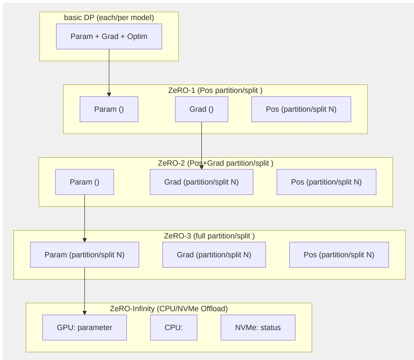
图13-9 DeepSpeed ZeRO 各阶段内存分布
