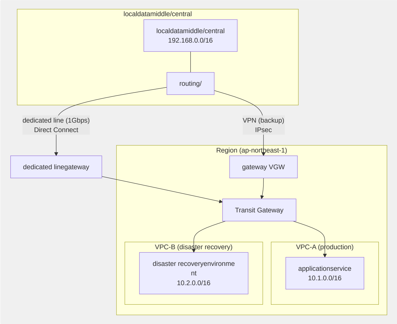
图7-7 混合组网架构：专线 + VPN 主备方案
