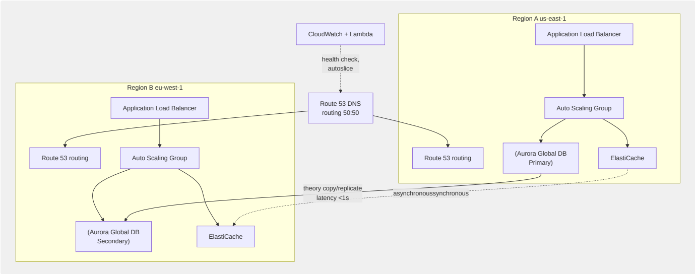
图18-12 Aurora Global Database 多 Region 双活架构
