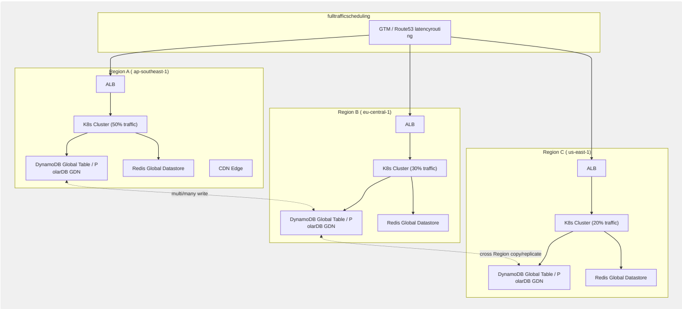
图C-6 全球多活架构
