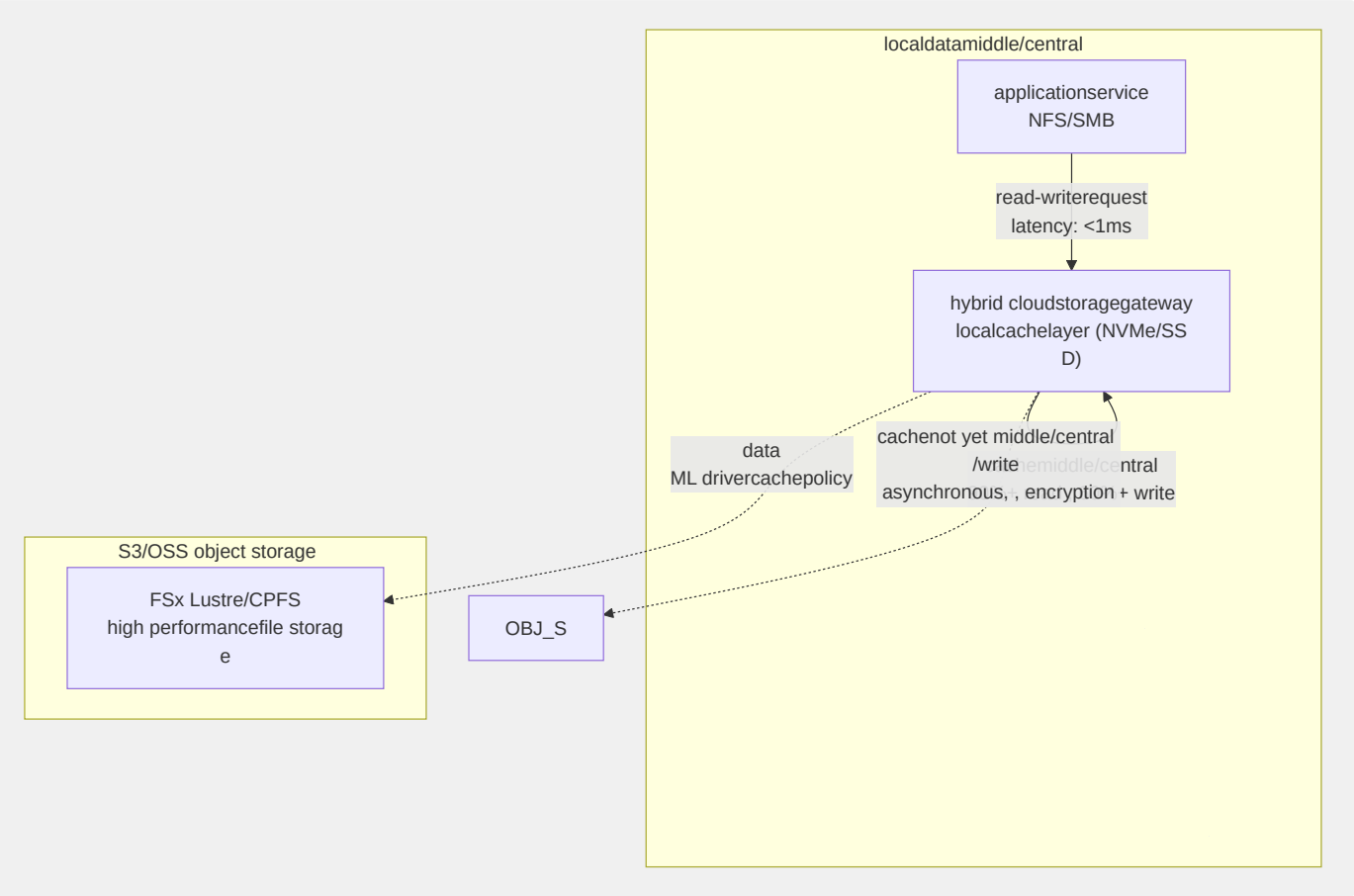
图6-19 混合云存储网关缓存加速架构
