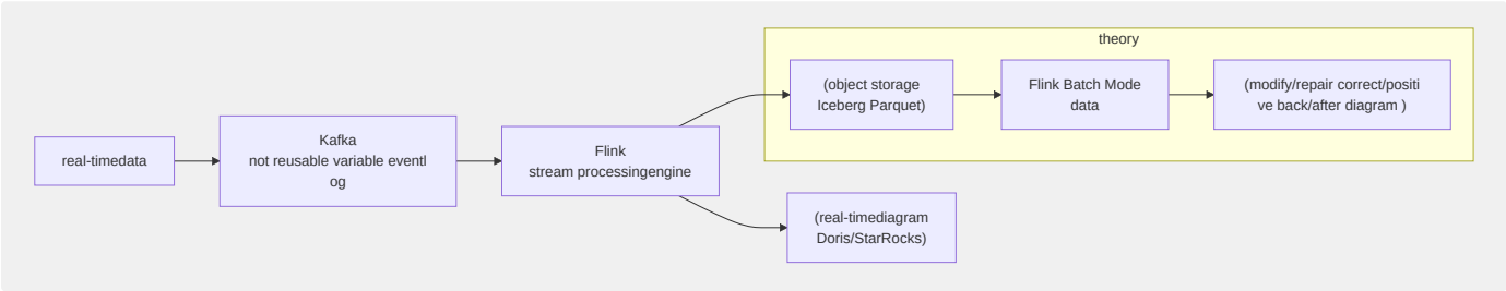
图12-14 Kappa 架构
