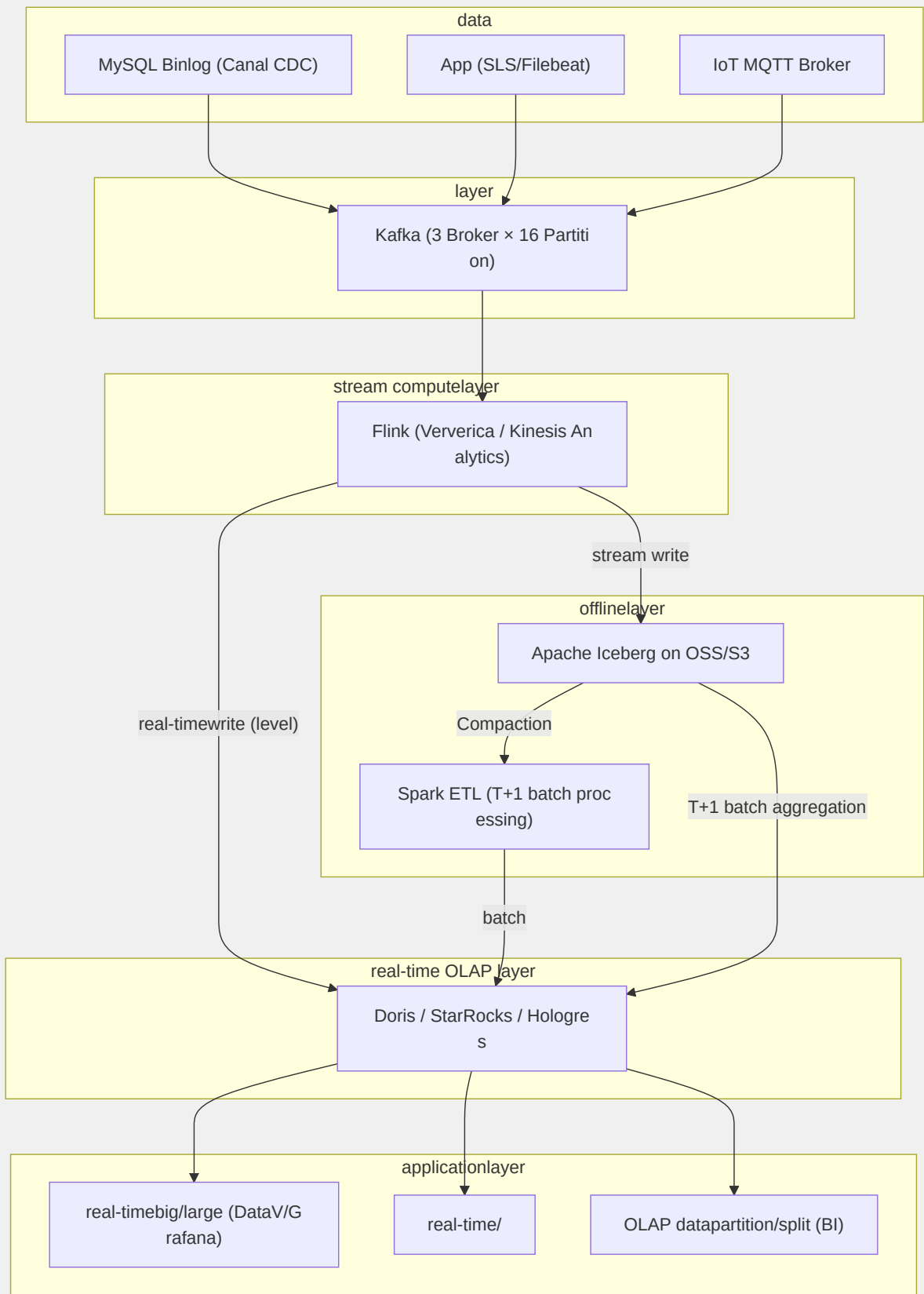
图C-3 实时数据处理架构
