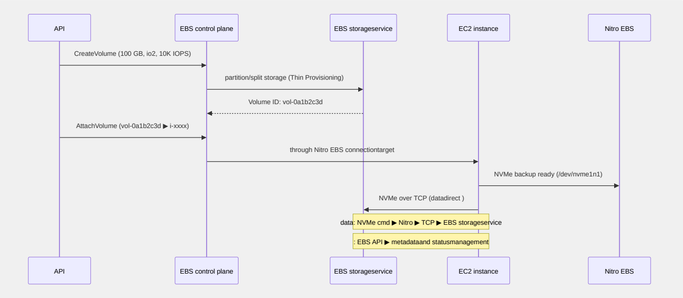
图6-7 EBS Attach 与数据通路
