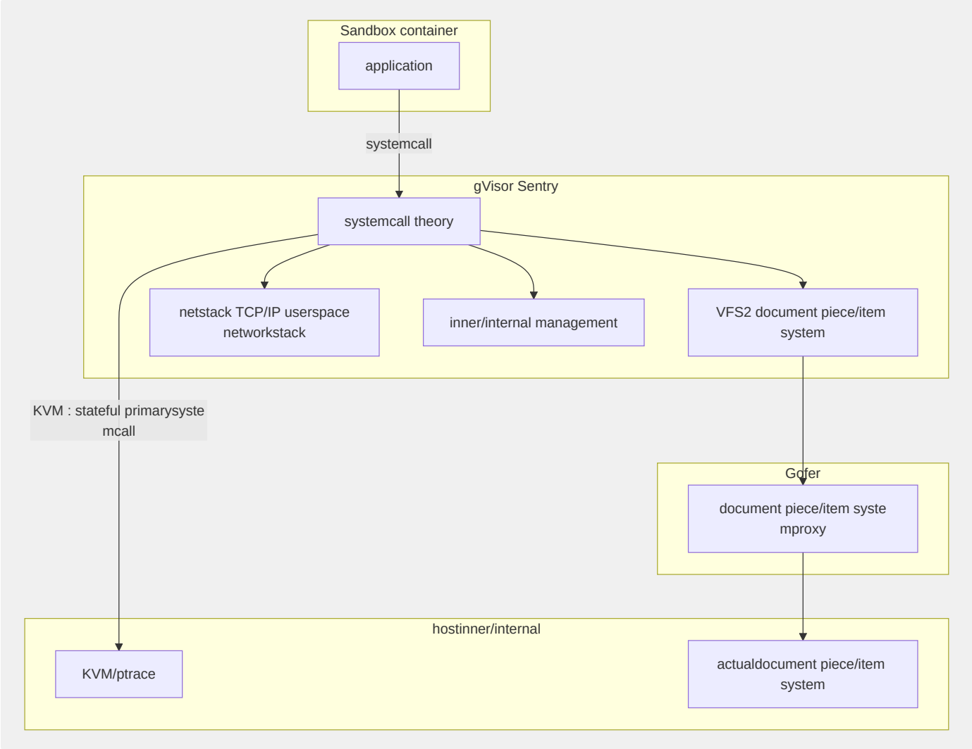
图8-7 gVisor Sentry 用户态内核架构
