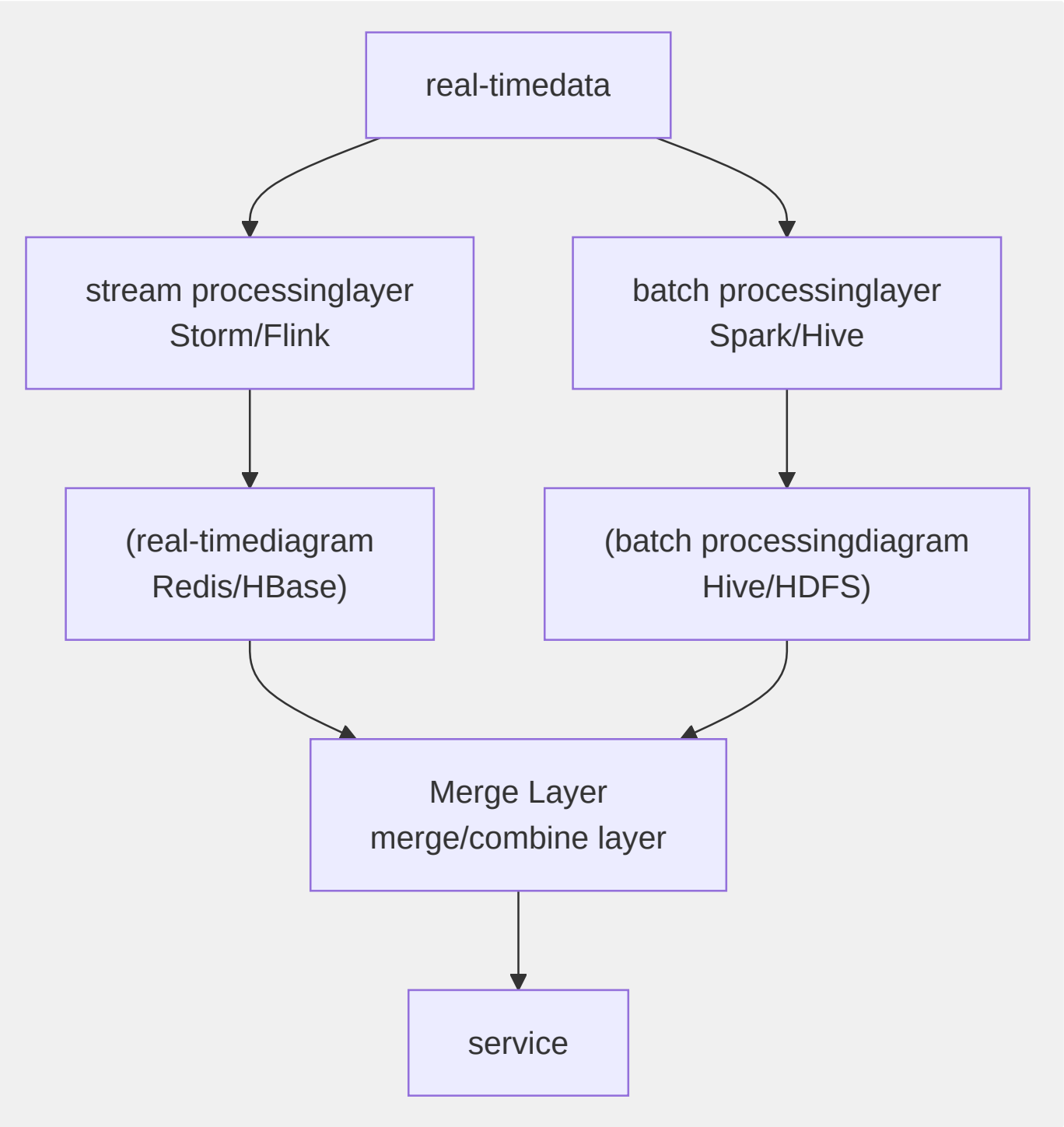
图12-13 Lambda 架构
