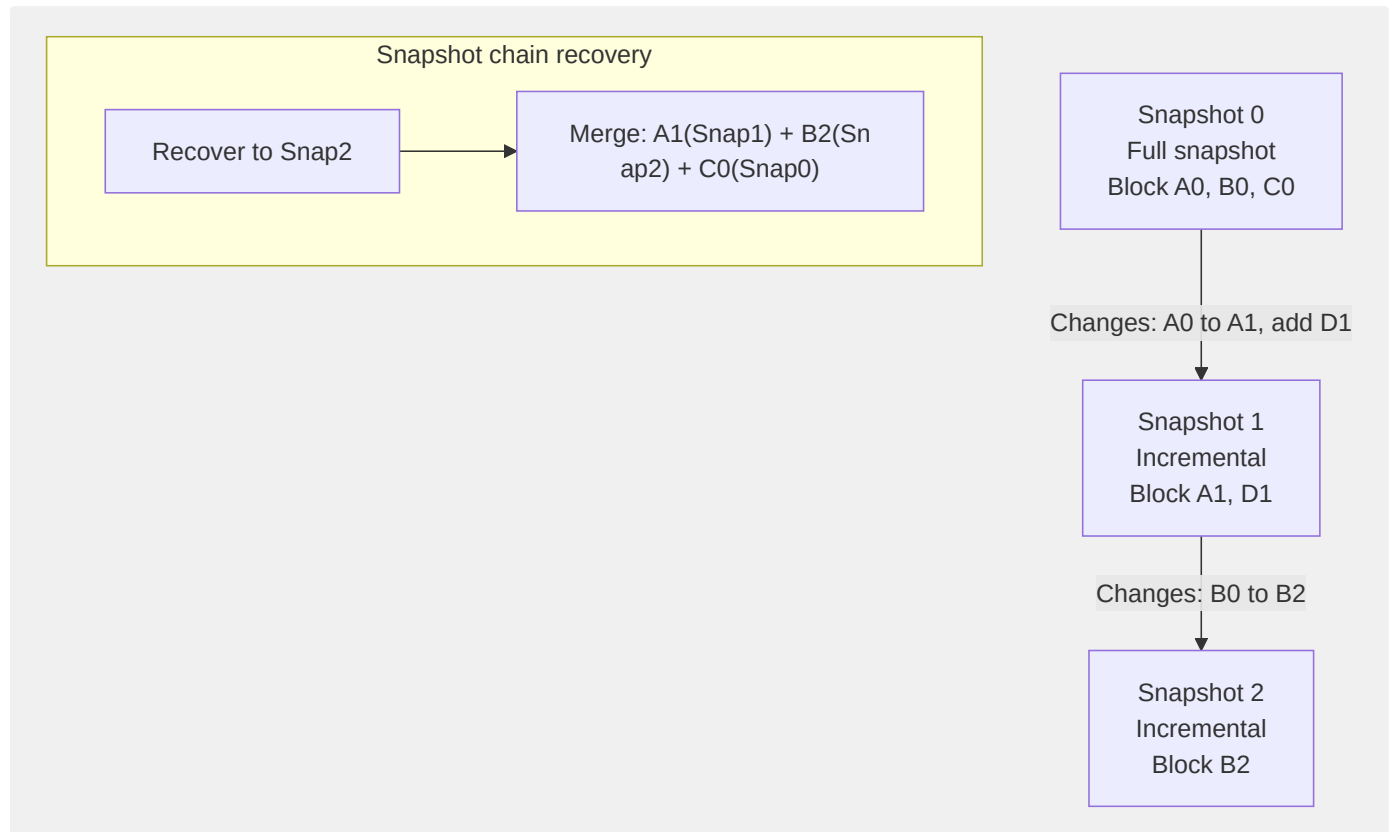
图6-8 增量快照链
