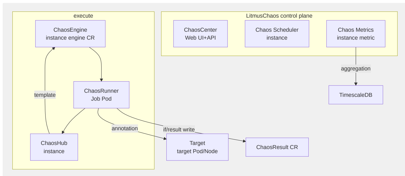
图16-14 LitmusChaos 架构
