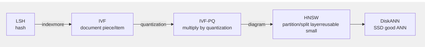
图11-5 ANN 算法的演进路径
