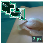
ShiftWM (ours)
