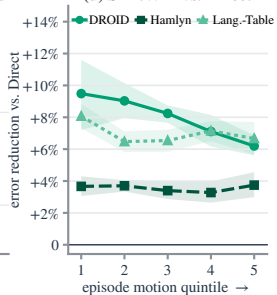
(d) ShiftWM vs. Direct
