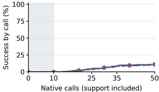
PushT
