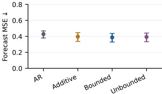
PushT
