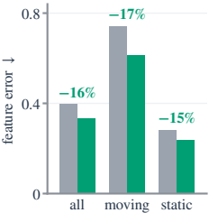
V-JEPA 2-AC, DROID test
