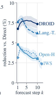
(d) At every horizon
