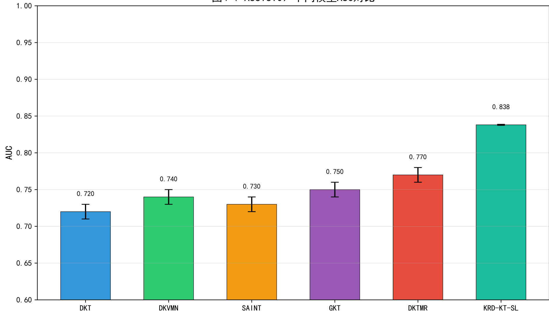
图4-1 ASSIST09 不同模型AUC对比
