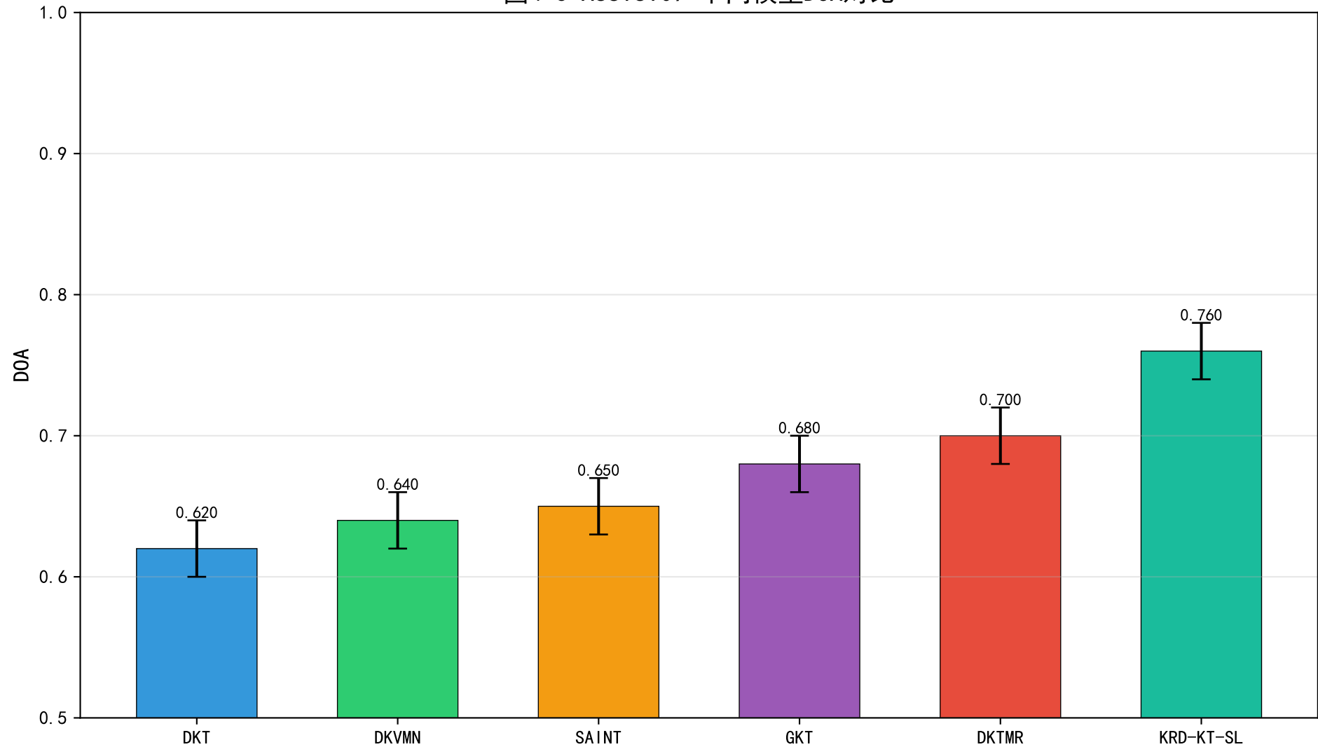
图4-3 ASSIST09 不同模型DOA对比
