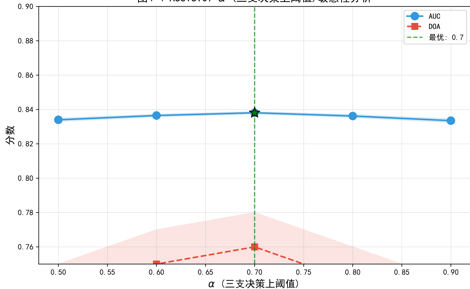
图4-4 ASSIST09 \alpha (三支决策上阈值) 敏感性分析
