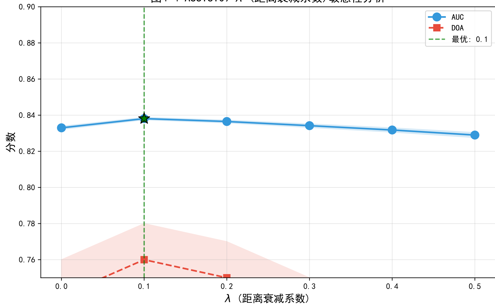
图4-4 ASSIST09 \lambda (距离衰减系数) 敏感性分析
