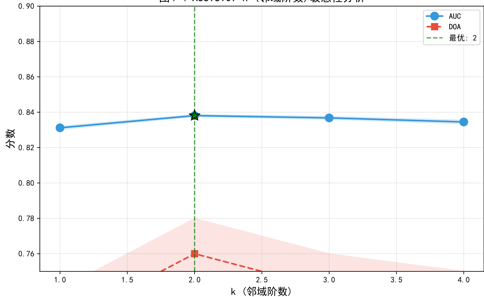
图4-4 ASSIST09 k (邻域阶数) 敏感性分析
