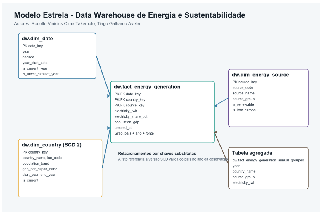
Figura 1 - Diagrama visual do modelo estrela
