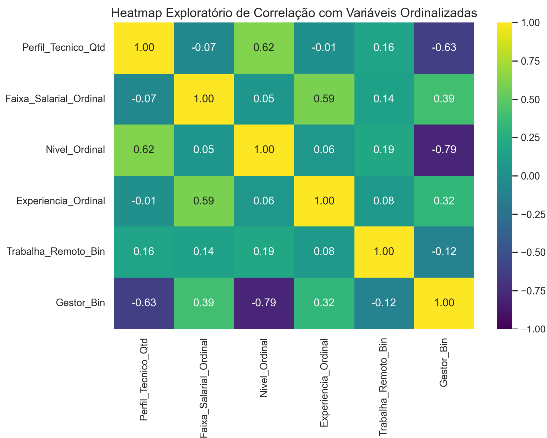
Figura 6 - Heatmap exploratório de correlação
