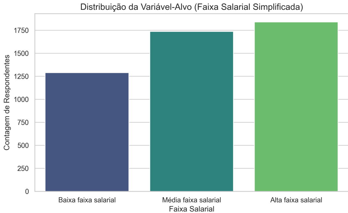
Figura 1 - Distribuição da variável-alvo simplificada
