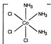
फलकीय समावयव (fac)
