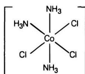
रेखांशिक समावयव (mer)
